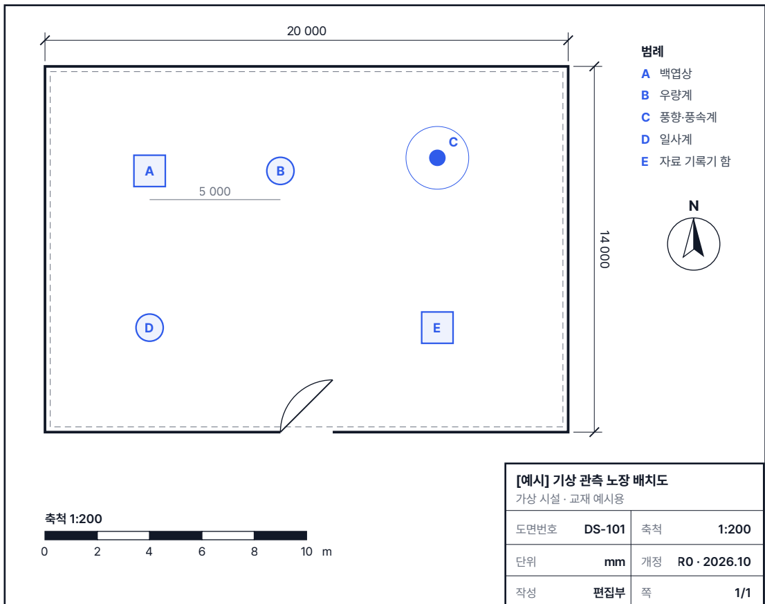
도면 1-1 가상 관측 노장 배치도(가상). 축척 1:200 (원도 1:100), 단위 mm, 도면번호 DS-101
